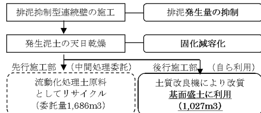
柱列式連続壁の泥土発生抑制と再利用
