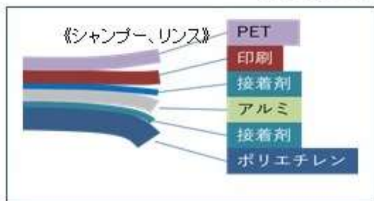
つめかえパックのフィルム断面図イメージ（例）
